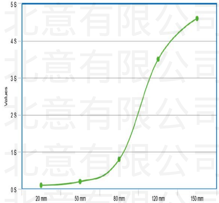
靜電消除距離與時間特性 ±1000 - ±100V
