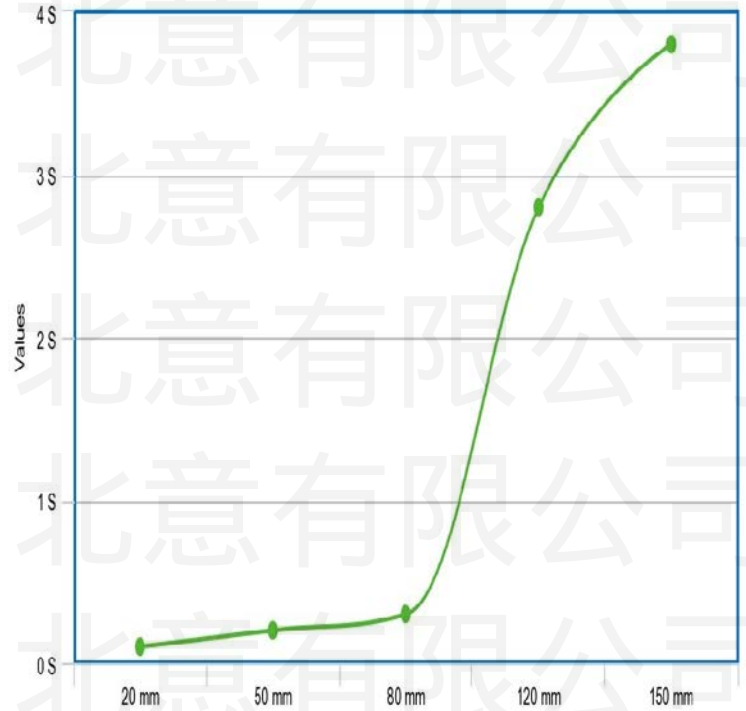
EC型靜電消除時間規格表(無氣源) 測試機型MODEL 280
